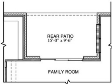
OPT. SLIDING DOOR UNIT
