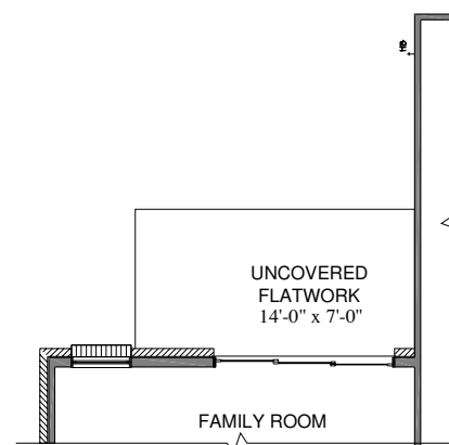
OPT. SLIDING DOOR UNIT
